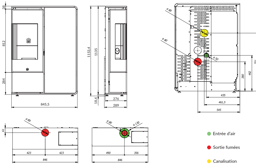
SORTIE FUMÉES CONCENTRIQUE INTÉGRÉE
