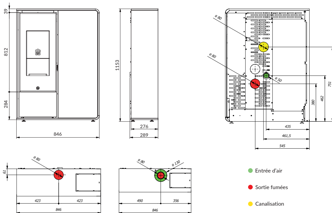
SORTIE FUMÉES CONCENTRIQUE INTÉGRÉE
